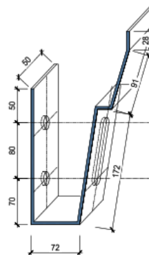
DETAIL KRYCEJ RÍMSY M 1: 5
