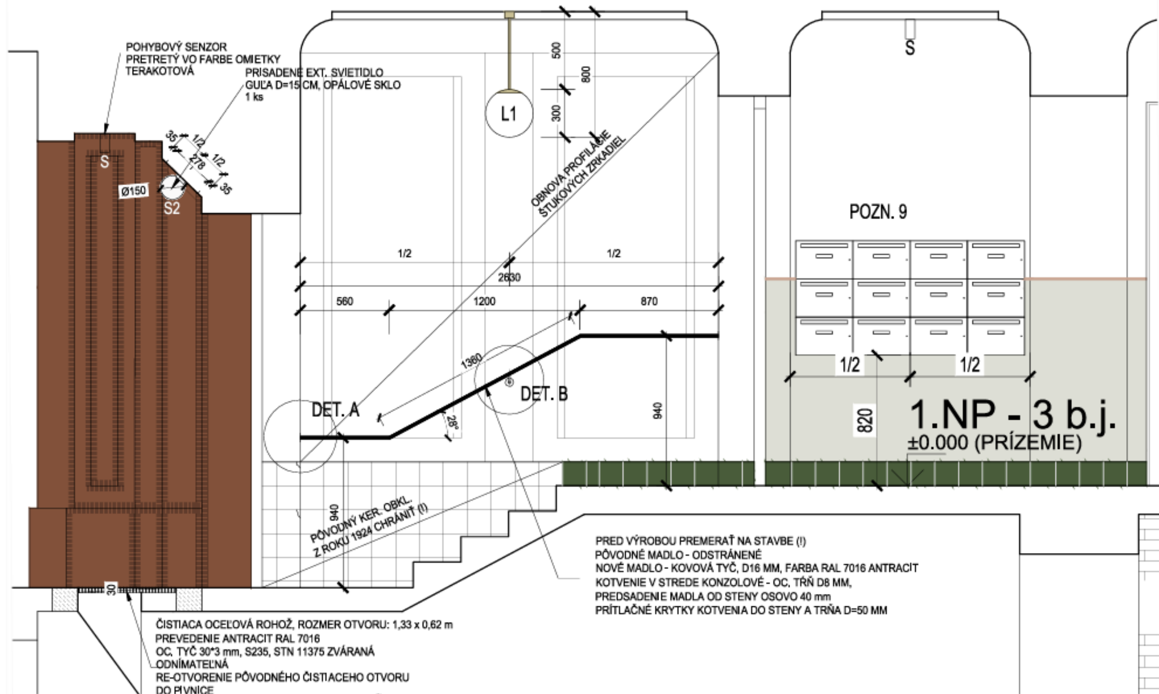
REZ VSTUPOM M 1:25
