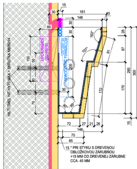
DETAIL KRYCEJ RÍMSY M 1: 5
