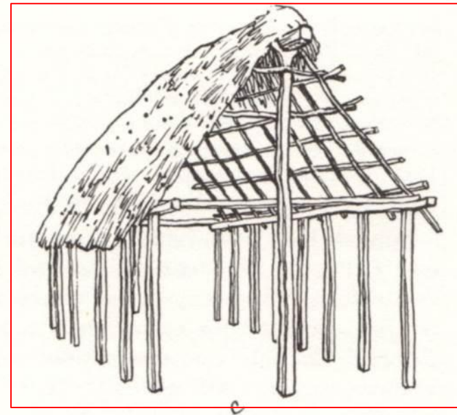
Sochový krov: a) Búč čp. 137, o. Komárno; b) Martovce c) Svätý Peter, o. Komárno
