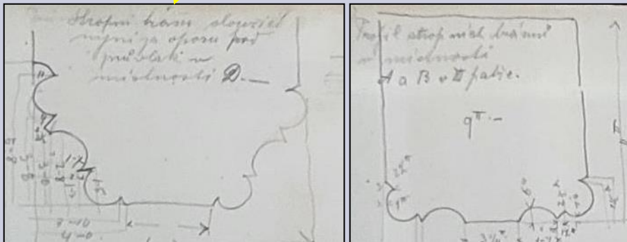
Profilované stropné trámy na 2. a 3. NP cisárskeho paláca (vľavo klinová forma, vpravo obdĺžnik/štvorec)
