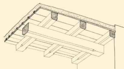
Priečne ukladané záklapové dosky s podopretím voči priehybu trámov kolmou mešternicou
