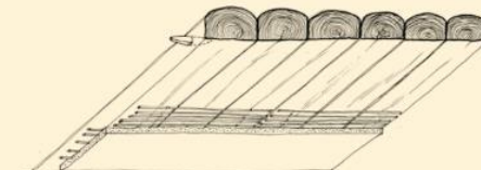
Príklad konštrukčného princípu povalového stropu
